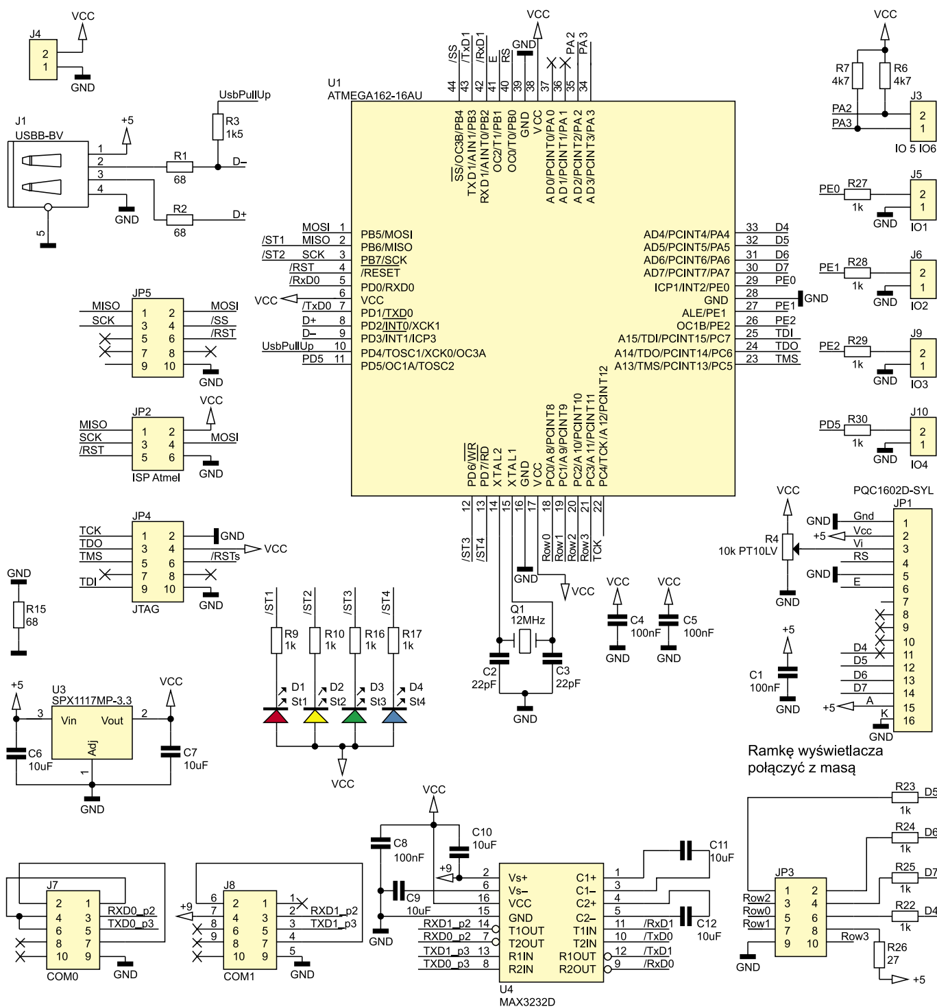
Rysunek 1. Schemat ideowy płytki testowej
